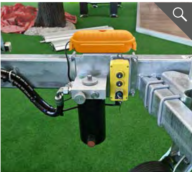
Sicherheitsbox (UDK mit Spinlock): Netzstecker und Steckschlüsseinsatz für die Notpumpe Pumplless
