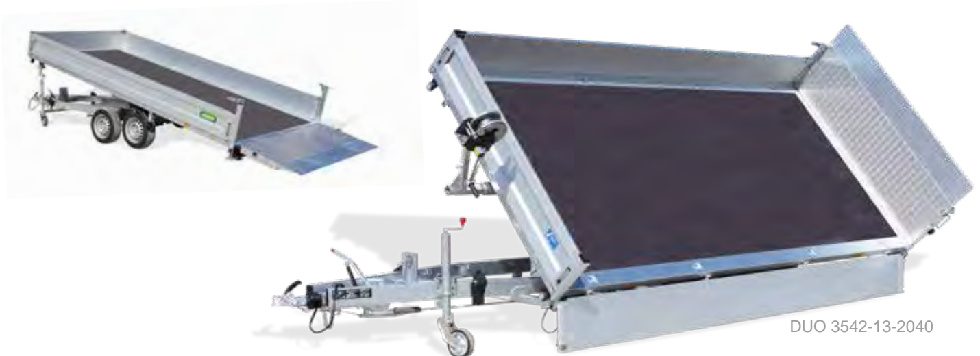
Durchgehende Stahlgitterauffahrklappe mit Alu-Riffelblech belegt
